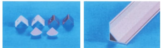
Model : HC - 013 Size : L x 17.35 x 6.9 PCB : 12mm
